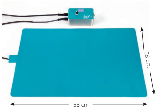
MCOI-445 Hot Mat 230 V / 50Hz
