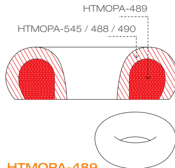
HTMOPA-489 INSERIMENTO Ø ext. 153 mm Ø int. 78 mm H 44 mm Vol: 520 ml 1 pc/pz
